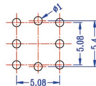
P.C.B LAYOUT
