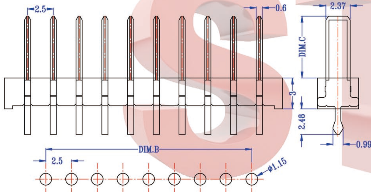
P.C.B LAYOUT
